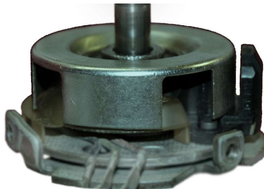
Foto: Für einen Motor mit 4 Zylindern wird ein Blendenrotor mit 4 Öffnungen benötigt .
